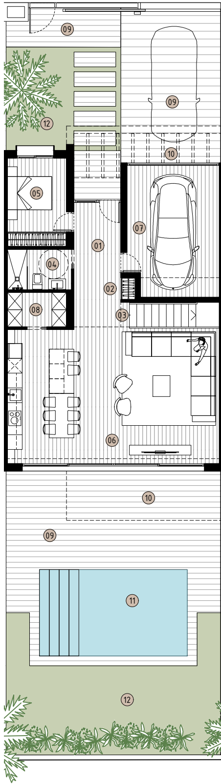
PARCELA 6: PLANTA BAJA
